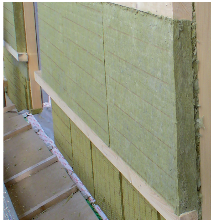
Abb. 6: Befestigung durch Klemmen
