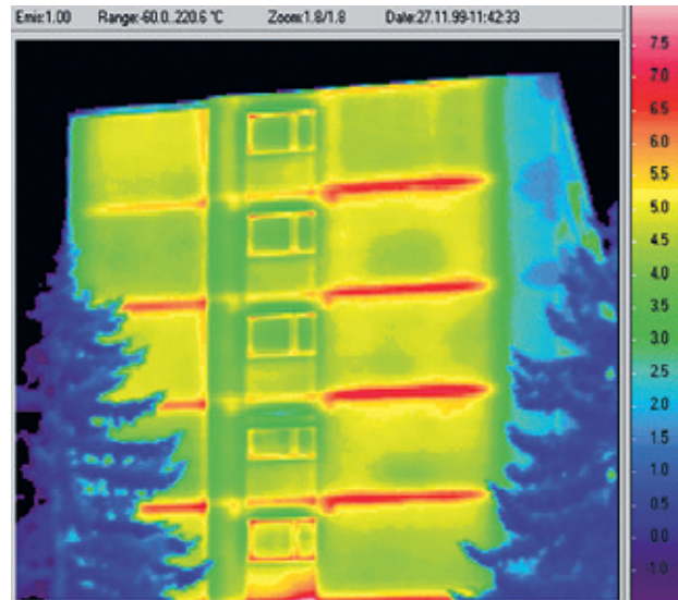
Un thermogramme permet de mettre en lumière les points faibles du bâtiment. Sur l'image, on voit clairement les déperditions de chaleur au niveau des plafonds (en rouge).
