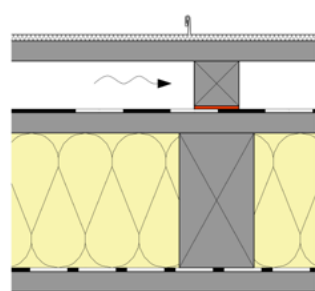
Abb. 5: Gegenüberstellung der beiden Systeme, eine homogene Verlegung sowie eine inhomogene Verlegung.
