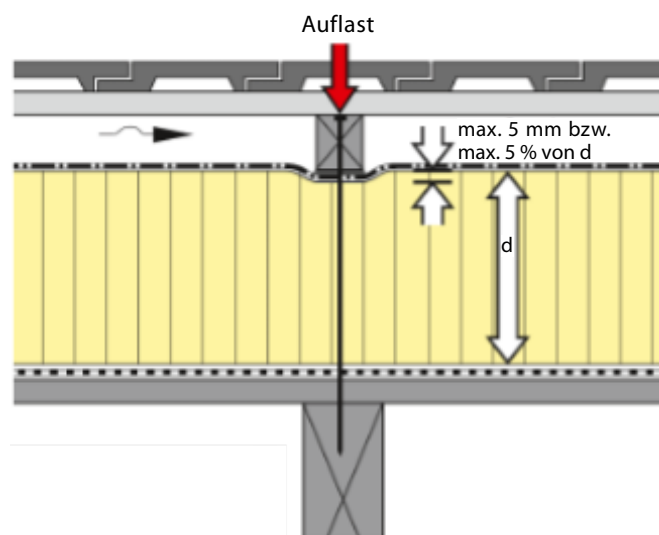
Abb. 7: Maximale Deformation von 5 % der Gesamtdicke oder maximal 5 mm.
