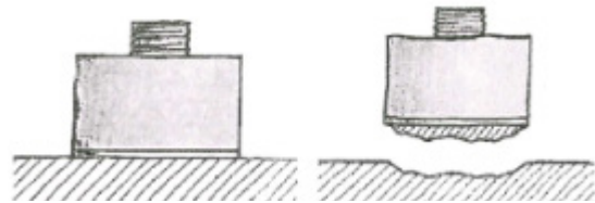
Abb. 1: Prüfung der Oberflächenzugfestigkeit z. B. von Beton
