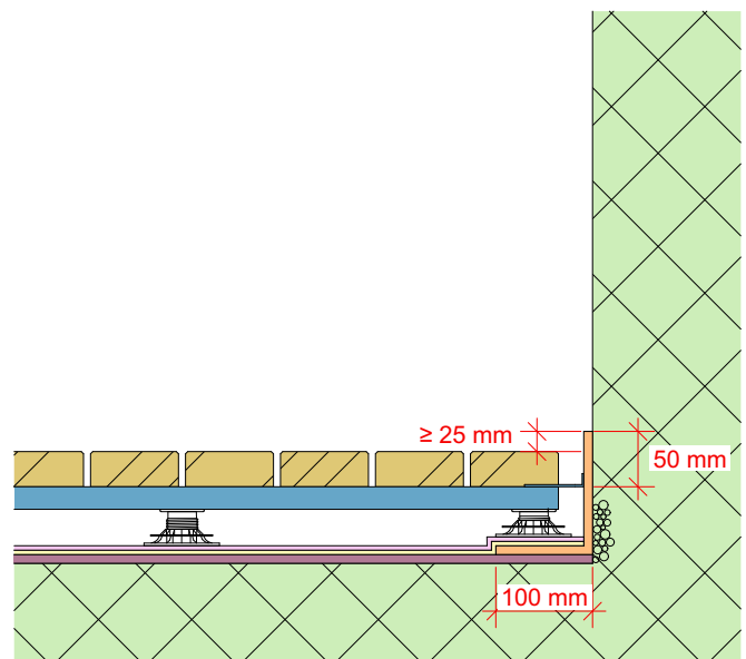
Abb. 8: FLK-Abschluss bei einlagigen Abdichtungen auf starre Untergründe. Anschlussfläche 50 mm ab festem Untergrund z.B. über einem Kiesnest.
