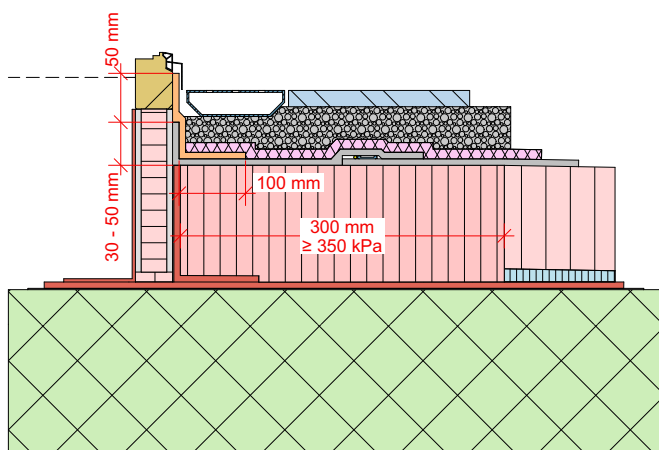
Abb. 10: FLK-Anschluss auf Abdichtung aus Kunststoff-Dichtungsbahn bei geschlossenen Nutzschichten, Anschlusshöhe der Abdichtung < 60 mm über Gehbelag/Nutzschicht
