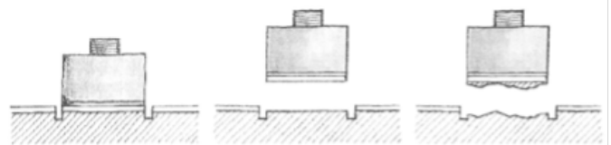
Abb. 2: Prüfung der Haftzugfestigkeit z. B. von FLK
