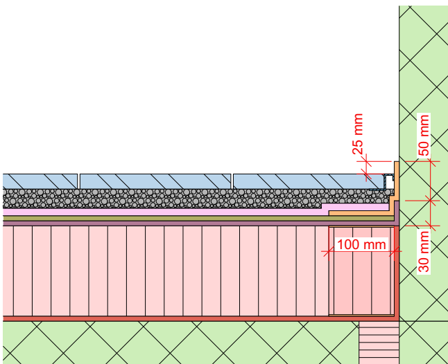
Abb. 6: Bei gedämmten Schichtaufbauten muss ein Dämmstreifen auf den Untergrund befestigt oder mit diesem verklebt werden.
