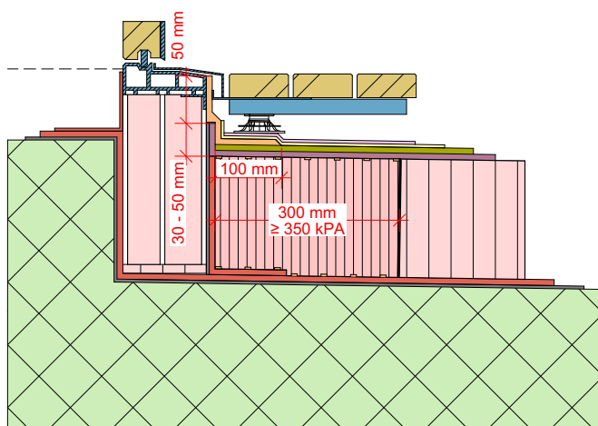
Abb. 9: FLK-Anschluss auf zweilagiger bitumiger Abdichtung bei Schwellenanschluss, Anschlusshöhe über Nutzschicht unter 60 mm.
