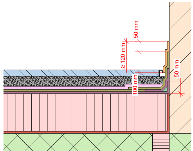
Abb. 7: Oberer Abschluss mit FLK als Ersatz des Blechabschlusses. Die bitumige Aufbordnung wird konventionell mit Keil und Eckverstärkung ausgeführt.
