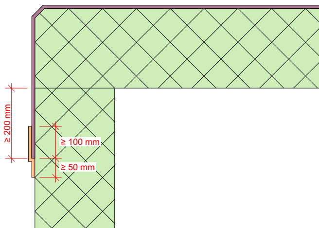
Abb. 11: Abbordung bei Abdichtungen unter Terrain nach Norm SIA 271
