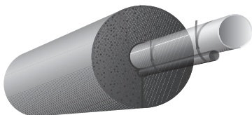
Ein effizientes Zirkulationssystem besteht aus einer Rohr-an-Rohr-Installation in gemeinsamer Wärmedämmung (grösseres Rohr als Vorlauf, kleineres als Rücklauf).
