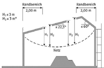
* Das Material der Schutznetze (Sicherheitsnetze) nach DIN EN 1263-1 ist für abstürzende Personen aus einer Höhe von maximal 6,0 m ausgelegt Abb. 1: Absturzhöhen für Schutznetze System S
