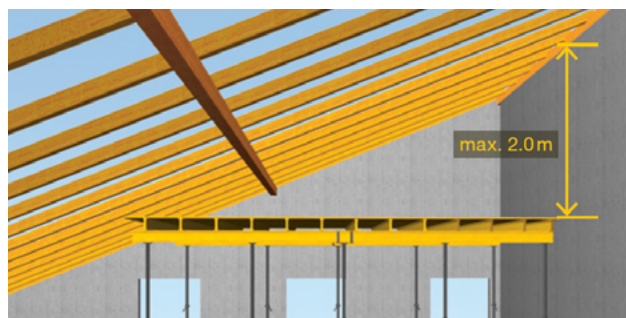
Fanggerüst unter einer Tragkonstruktion
