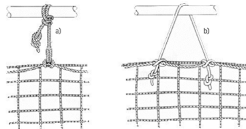
a) einsträngigem Aufhängeseil L (Seil-Bruchkraft ≥ 30 kN) b) zweisträngigem Aufhängeseil Z (Seil-Bruchkraft ≥ 15 kN)
