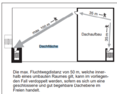
Abbildung 408-11: Maximale Fluchtwegdistanzen auf Dachflächen
